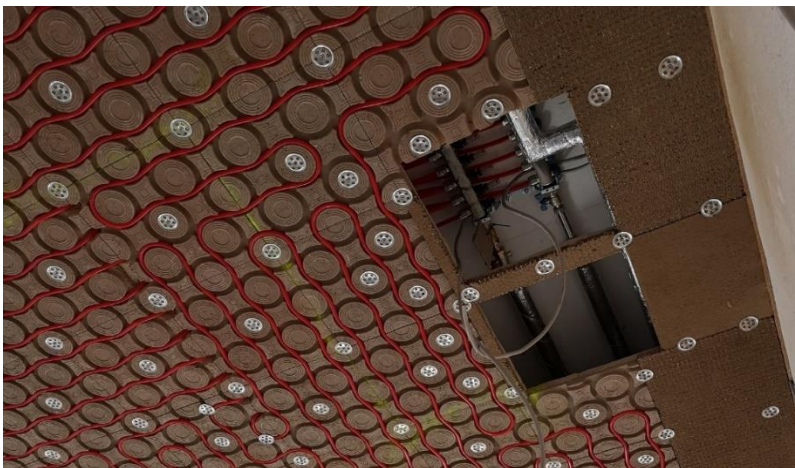
Positionierung des Heizkreisverteilers in der Zwischendecke.
